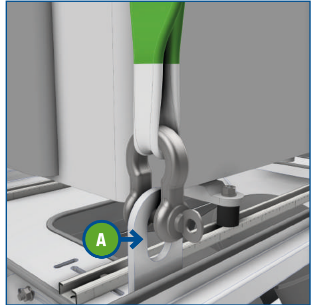
Figuur 2: Detail verbinden hijsonderdelen
